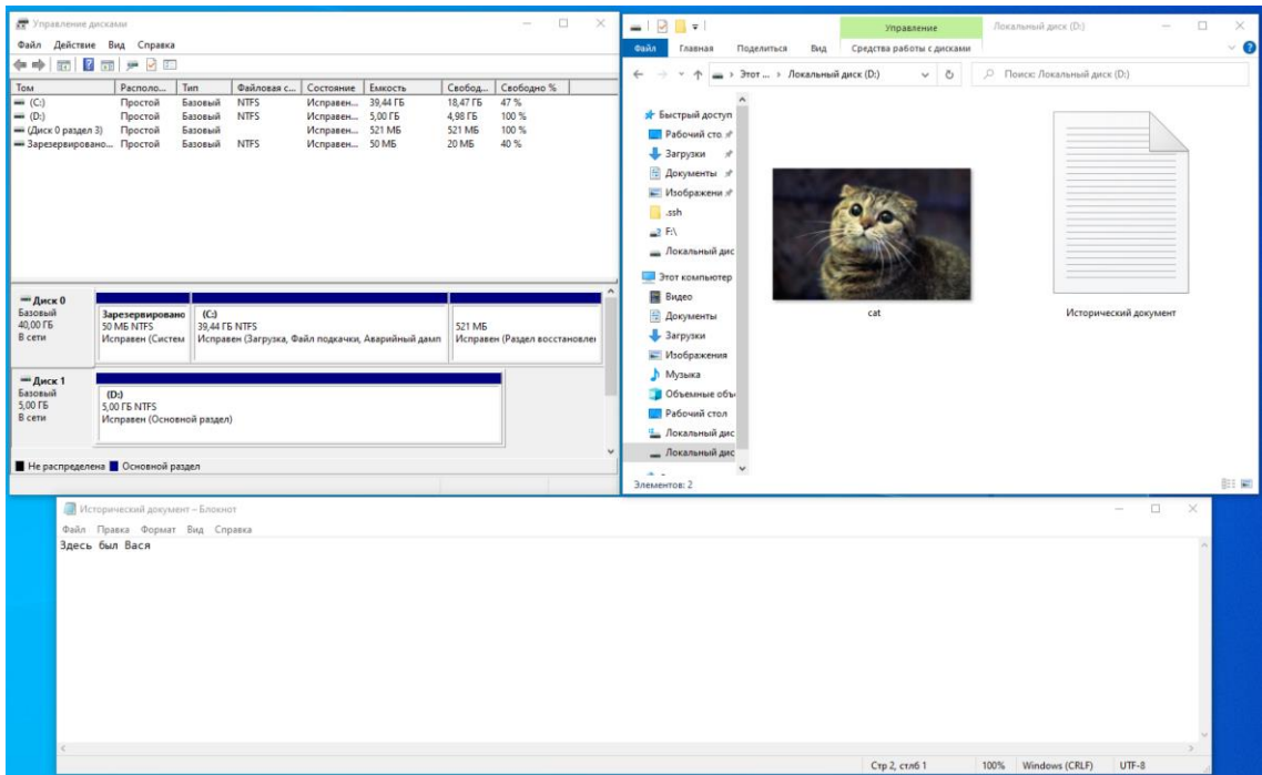
Рисунок 12. Проверка работы
