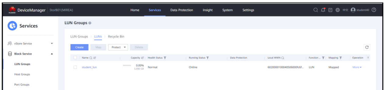
Рисунок 2. Созданный LUN
