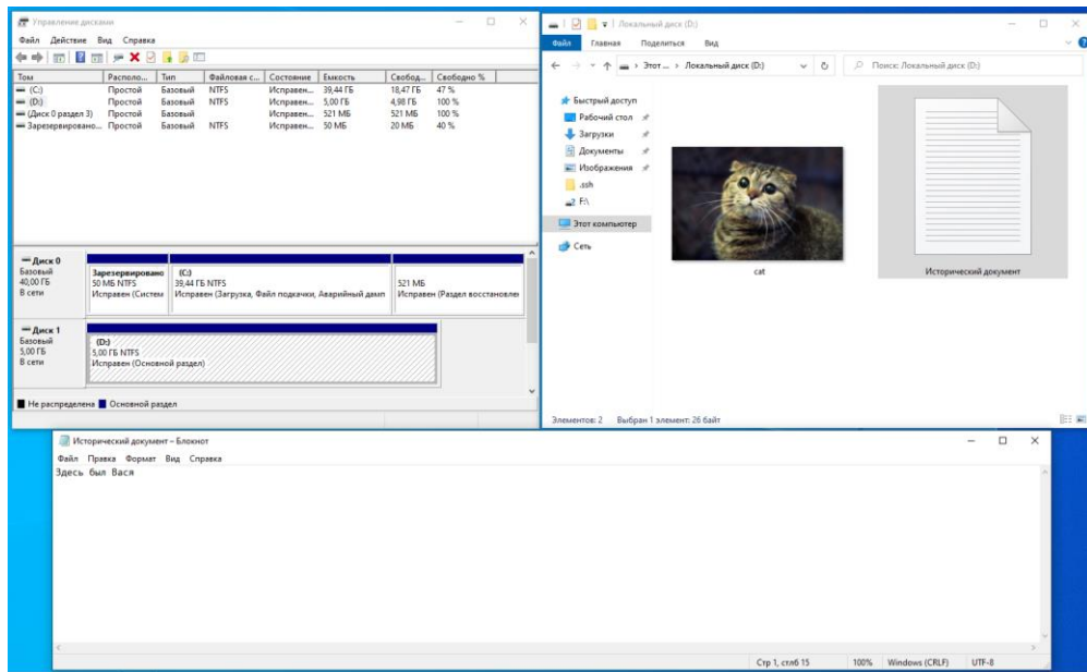
Рисунок 6. Заполненный том
