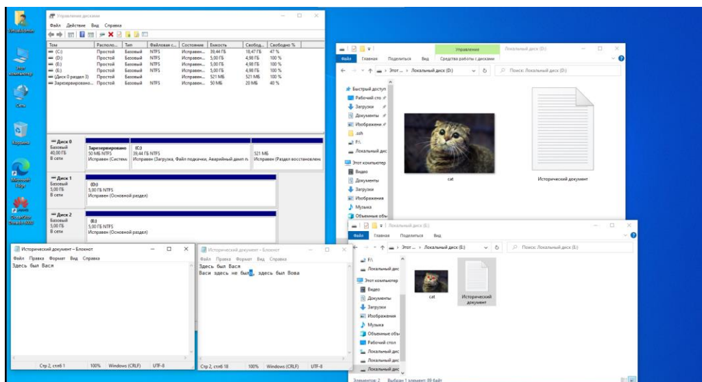
Рисунок 13. Итоговая проверка
